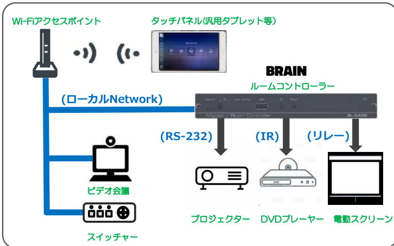
BRAIN内蔵のルームコントローラー（ゲートウェイ機能付き）を配置し BRAIN機能と信号変換を同時に行います
